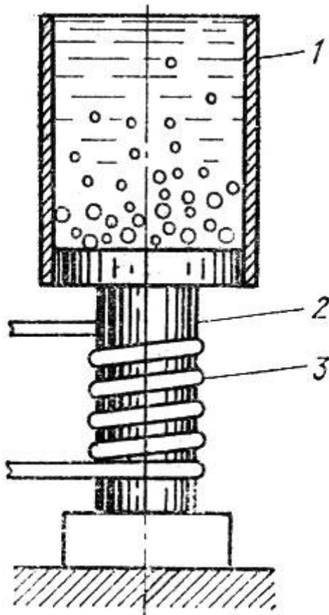
Рис. 5. Схема для кавитационной обработки деталей. 1 - ванна; 2 - сердечник; 3 - соленоид
