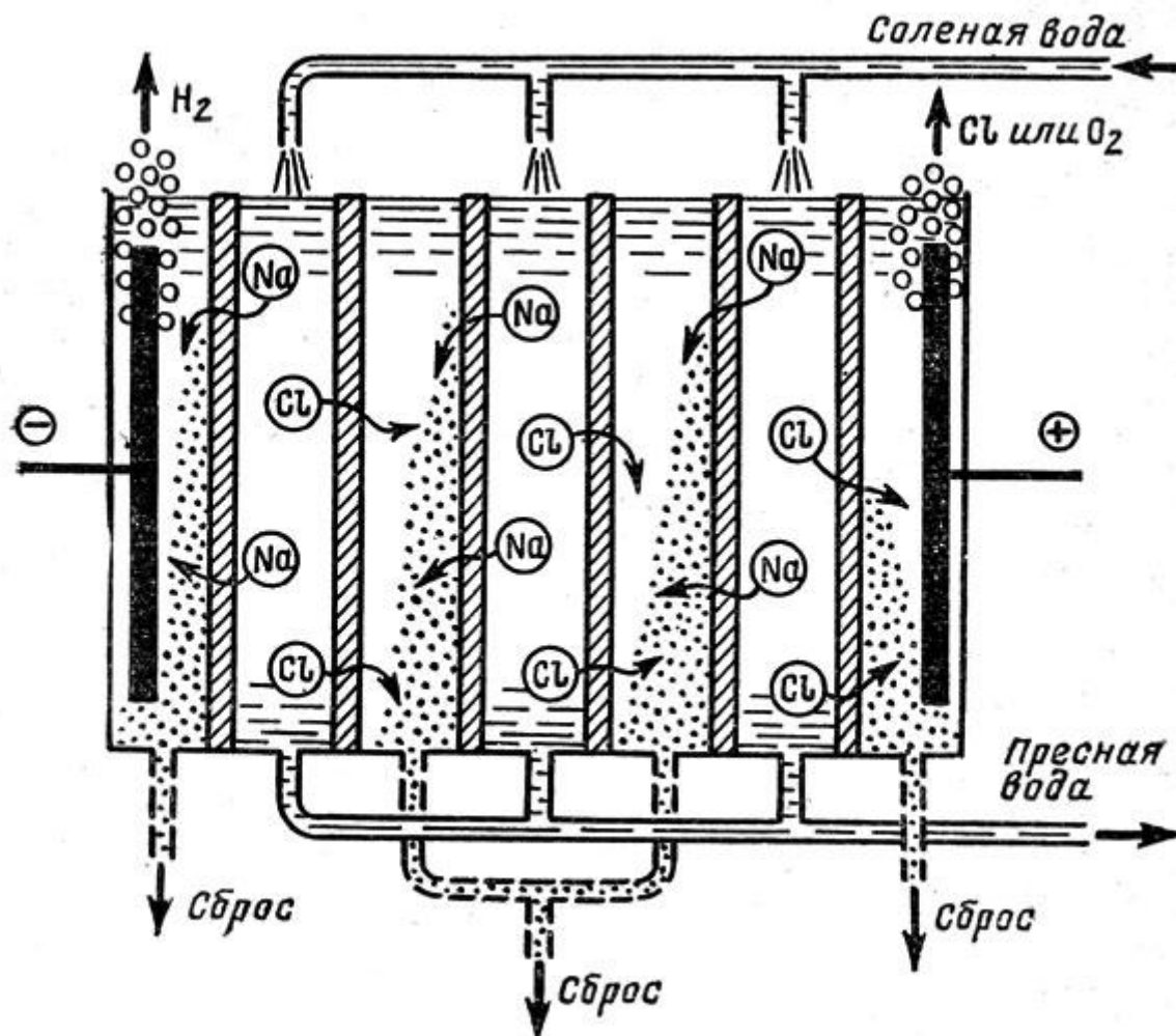
Рис. 3. Схема работы многокамерного электродиализатора
