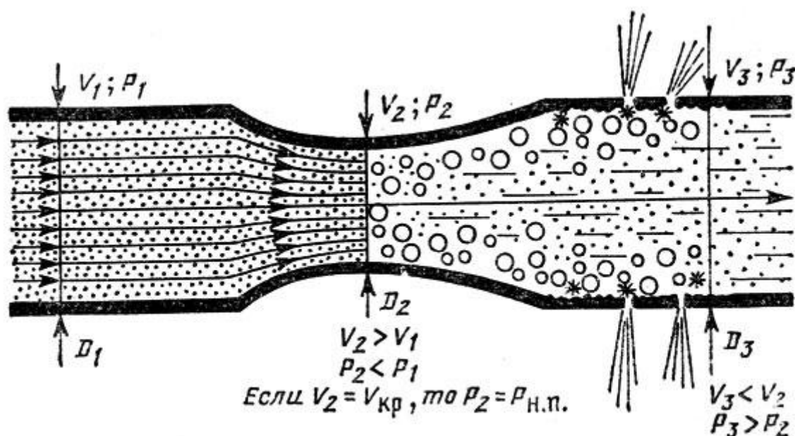
Рис. 4. Возникновение кавитации в трубопроводе
