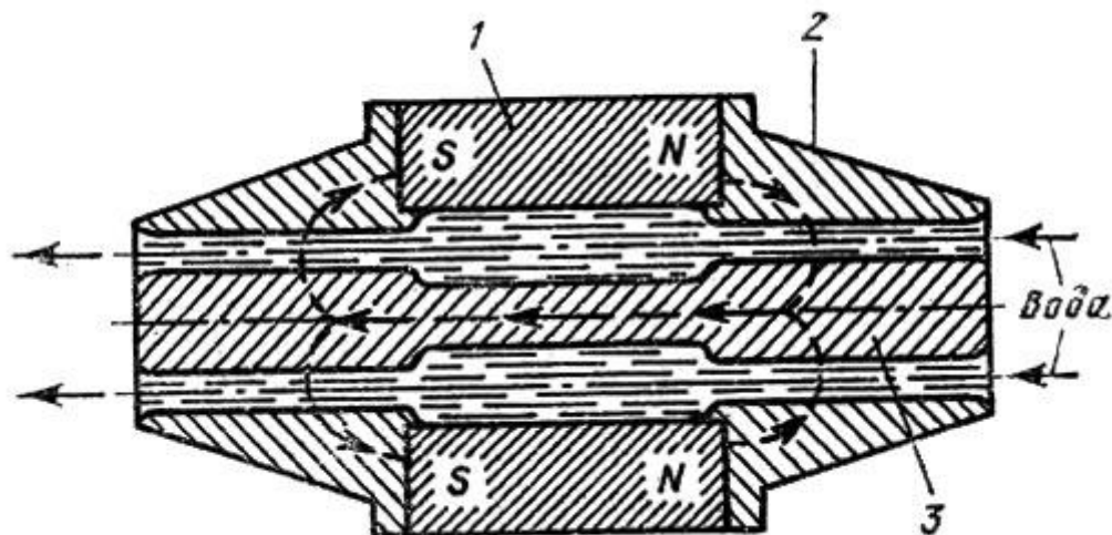
Рис. 8. Схема магнитной обработки воды. 1 - постоянный магнит; 2 - полюсные наконечники; 3 - сердечник
