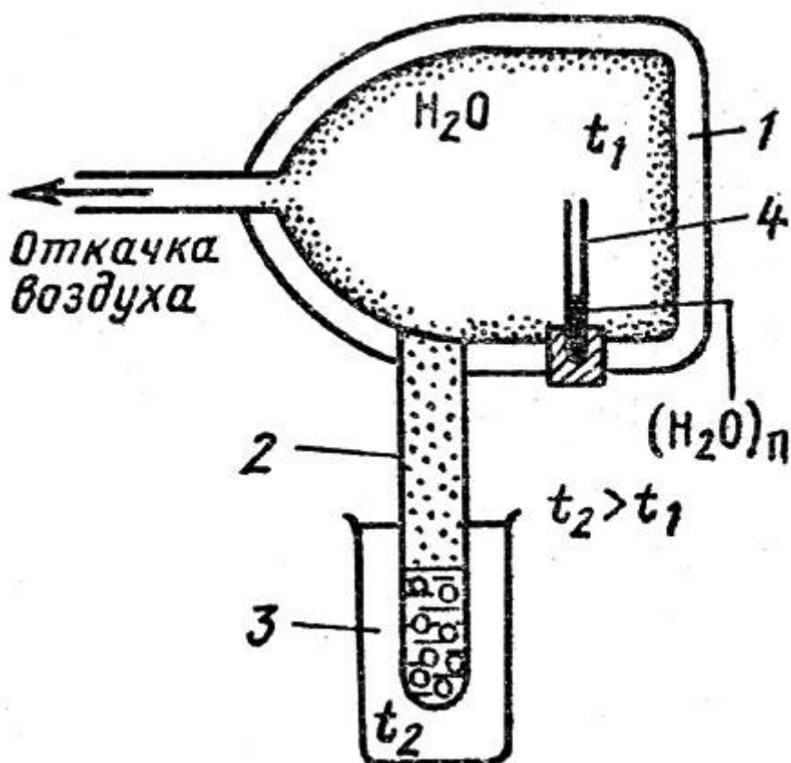
Рис. 7. Схема установки для получения воды II. 1 - сосуд Дьюара; 2 - пробирка; 3 - термостат; 4 - капилляр
